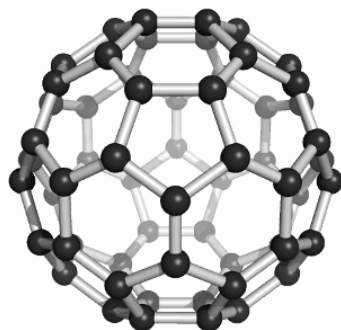
Эмблема НОЦ «АВТех» – фуллерен C_{60} .
